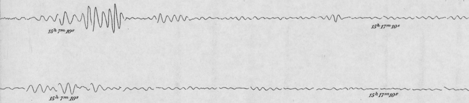
Fig. 7—8. Bodenschwingungen durch Glockengeläute (ab), normaler Verlauf der Registrierlinie (cd).
