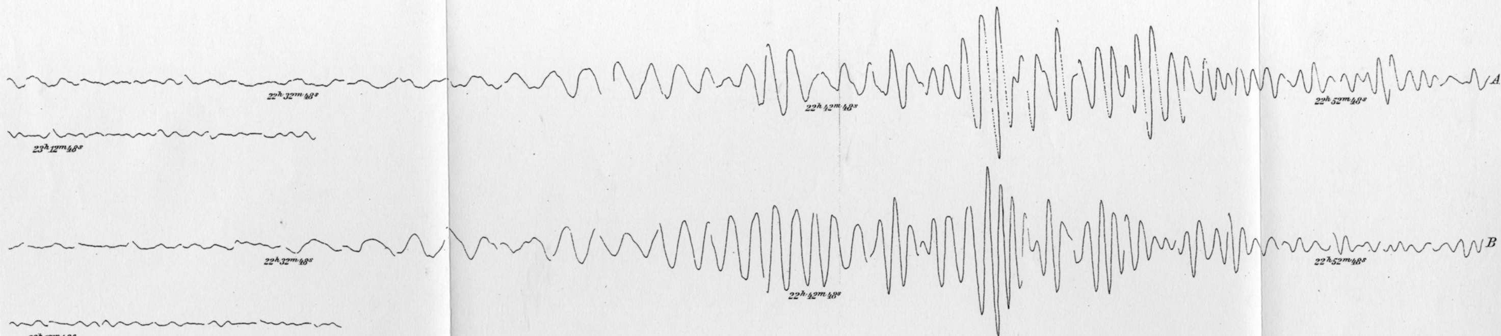
5-6. Seismogramme des Skandinavischen Bebens vom 23. Oktober 1904. 1. Einsatz 11 h 29 m 8 s
